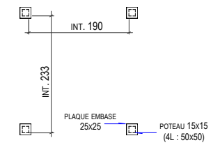
DÉTAIL D'IMPLANTATION DES POTEAUX SOUS-SOL ECH: 1CM = 1M
